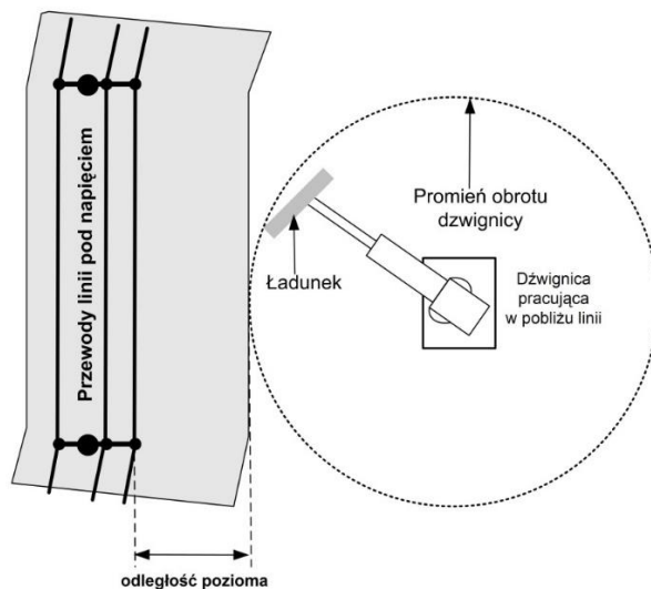
Rys 1. Strefa działania dźwignicy
